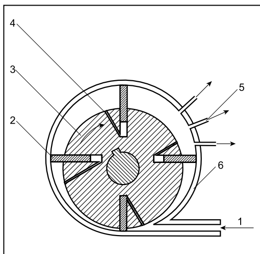
14.3 Zasada działania pneumatycznego silnika łopatkowego 1 – wlot sprężonego powietrza z mgłą olejową, 2 – łopafka, 3 – wirnik, 4 – otwory umożliwiające ruch łopatek, 5 – wylot rozprężonego powietrza, 6 – korpus silnika
