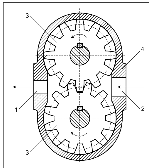
14.4 Zasada działania pneumatycznego silnika zębatkowego
